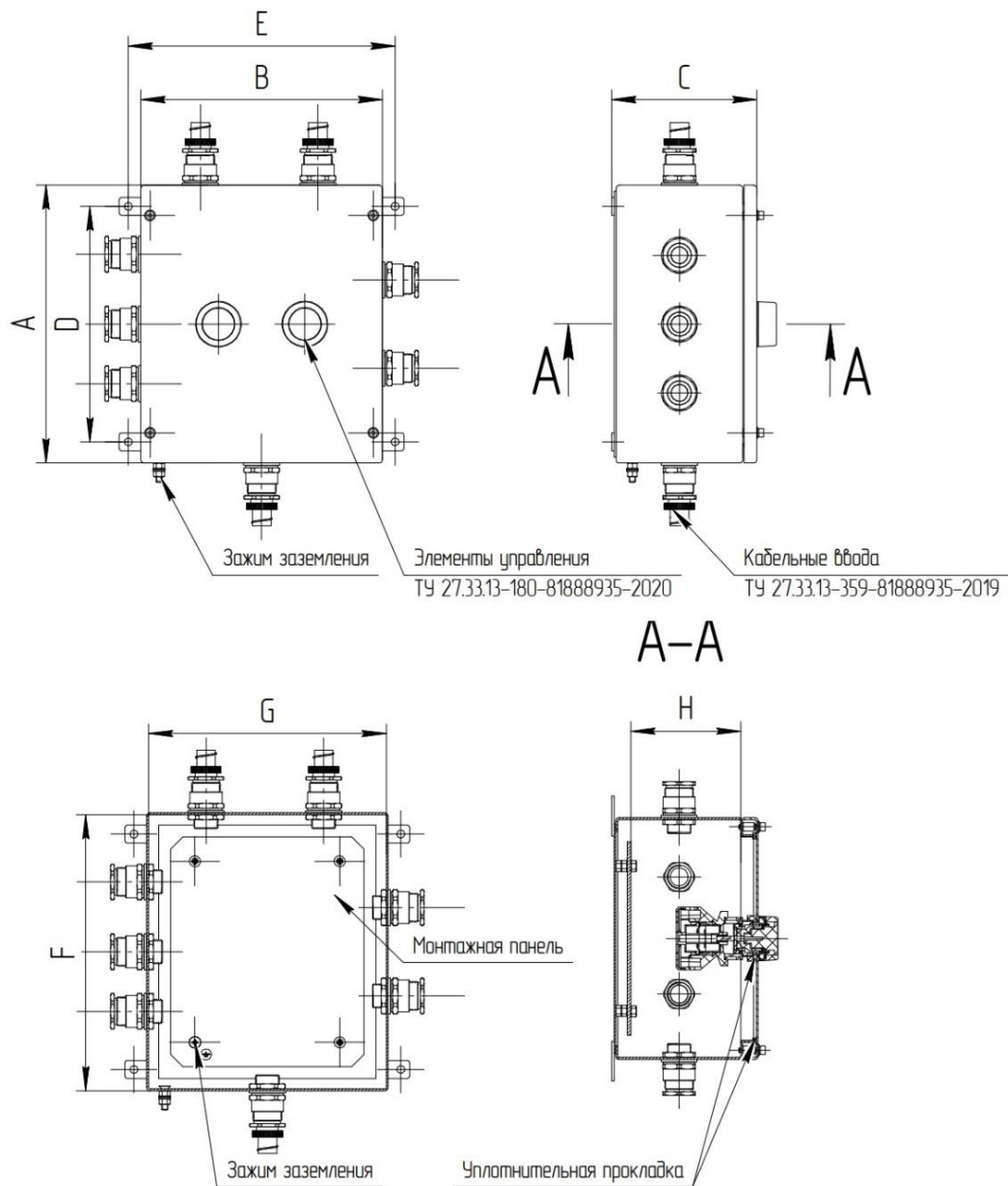
Рис.А1. Конструкция постов управления общепромышленных моделей ПКВ ОП-Н-XXX...X
