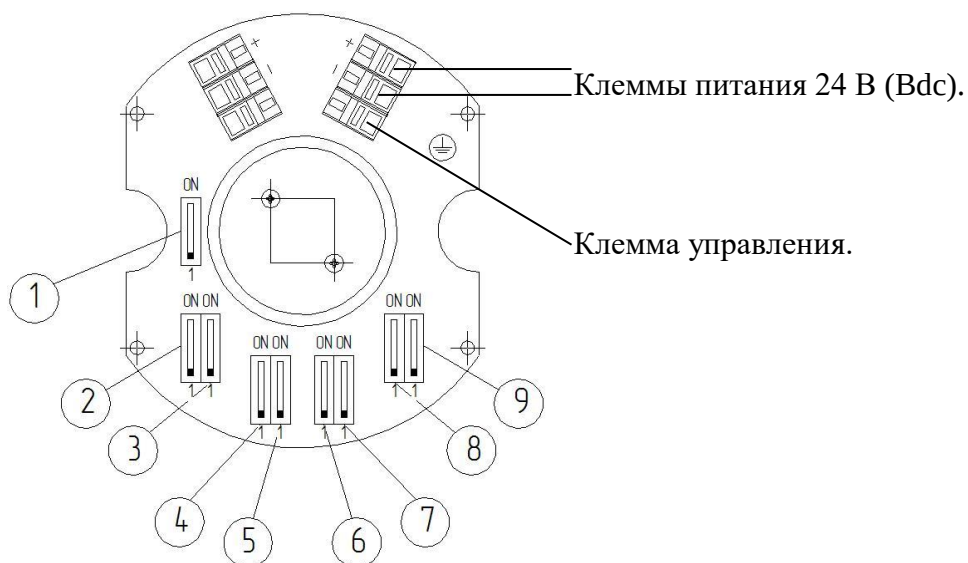
Рис. 1 Схема расположения элементов управления на печатной плате.
